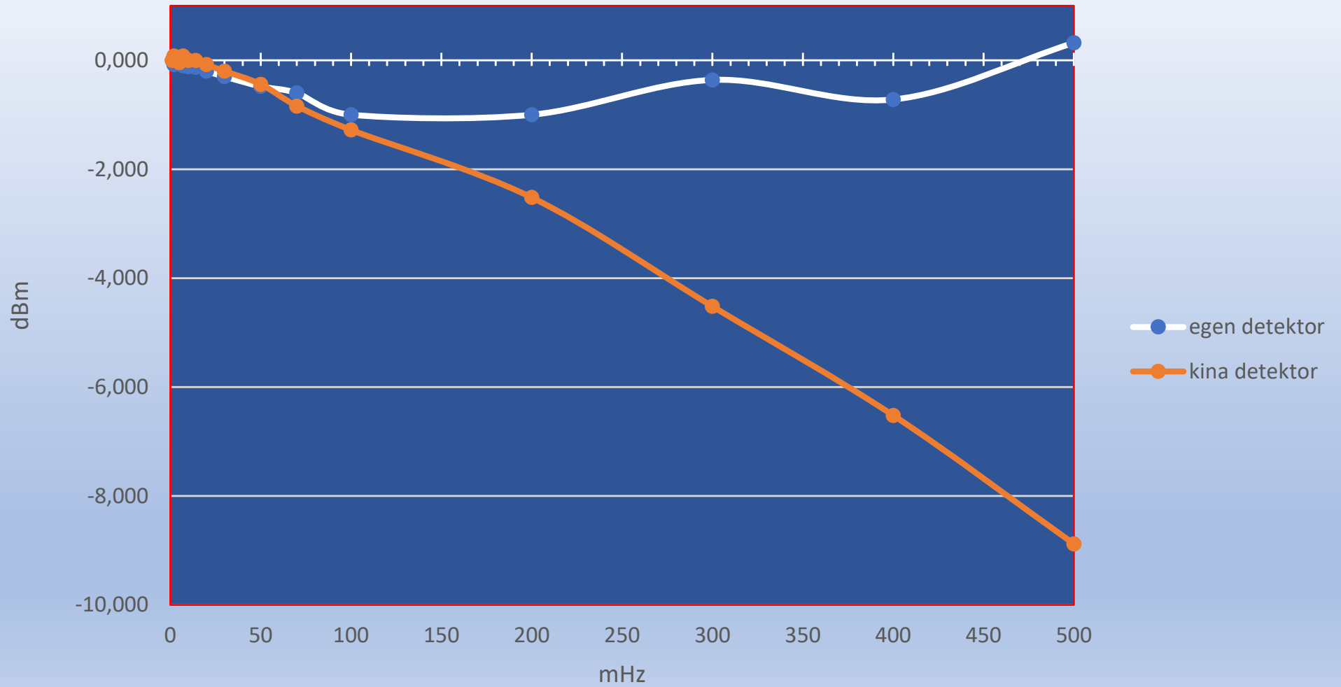
frekvensgang for egen detektor og kina-detektor
